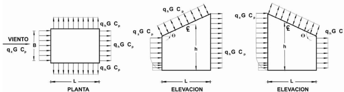
CUBIERTAS DE PENDIENTE ÚNICA (NOTA 4).
